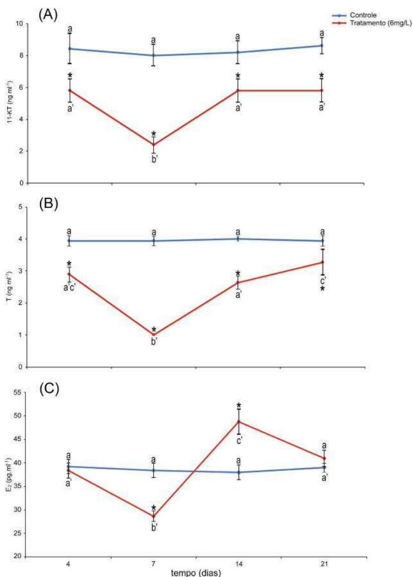
Figura 5. Níveis plasmáticos de: A) 11-Cetotestosterona (110KT); B) Testosterona (T); e C) 17β-Estradiol (E 2 ) (média + desvio padrão) em machos em ambos os grupos experimentais: controle (n=20/grupo), tratado 6mg/L (n=20/grupo) durante os 21 dias de exposição ao EDS. Grupos marcados com asterisco (*) denotam diferenças significativas ( p < 0.05 ) em relação ao grupo controle. Letras diferentes denotam diferenças significativas ( p < 0.05 ) dentro do mesmo grupo experimental.
