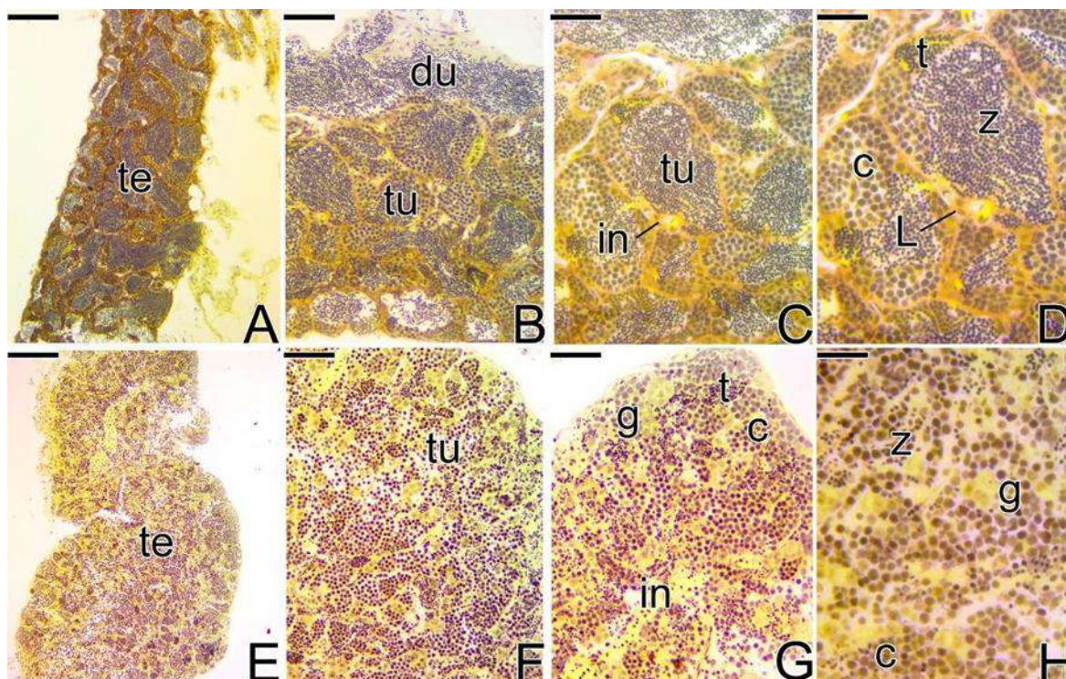
Figura 1. Cortes histológicos dos testículos de zebrafish comparando o Grupo Controle (A-D) e o Grupo Experimental 6mg/L (E-H) no 4ºdpe. A) Visão geral do testículo. B) Presença de espermatozoides no ducto espermático e nos túbulos testiculares. C-D) Túbulo testicular com lúmen preenchido por espermatozoides. Notar o epitélio germinativo definido, com espermatocistos, e compartimento intersticial delimitado, com presença de células de Leydig. E) Visão geral do testículo tratado. F-G) Túbulos testiculares pouco organizados. H) Túbulos testiculares desorganizados, com lúmen não definido. Espermatozoides escassos e interstício mal definido. Testículo (te), túbulos testiculares (tu), ducto espermático (du), interstício (in), espermatozoides (z), espermatócitos (c), espermátides (t), células de Leydig (L), espermatogônia (g). Coloração: Metanil Yellow. Barra: 100µm (A,E), 50µm (B,F), 30µm (C,G), 20µm (D,H).
