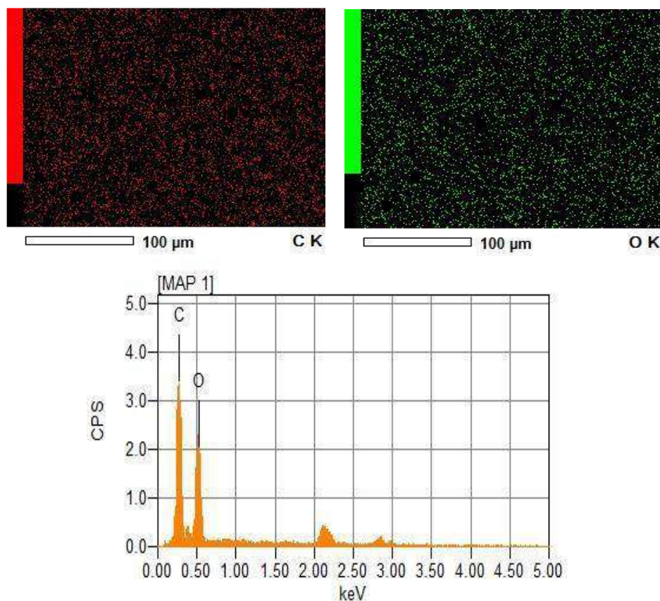
Figura 3. Espectro de EDS e imagens da amostra de quitosana indicando vermelho para carbono e verde para oxigênio.
