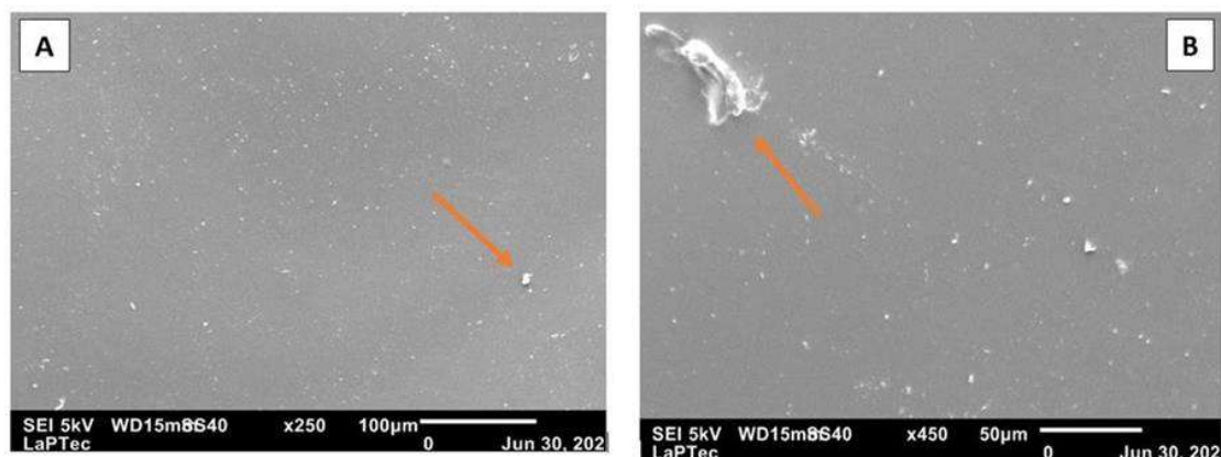
Figura 2. Imagens de MEV do filme de quitosana (A) Magnificação 250x, (B) Magnificação 450x.
