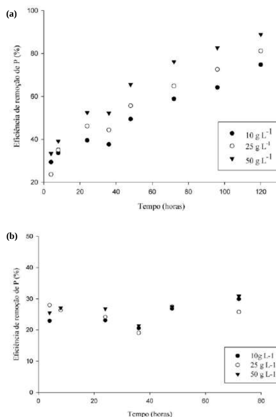
Figura 2. Eficiência na remoção de P pelos sacos adsorvedores de fósforo preenchidos com lodo da estação de tratamento de água (a) e com casca de ovo da galinha (b).
