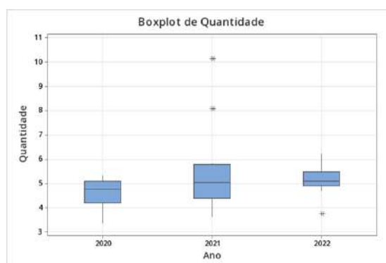
Figura 2. Gráfico Boxplot das amostras consideradas.
