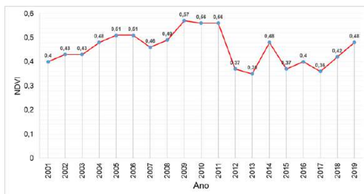
Figura 2. Série temporal da média anual de NDVI.
