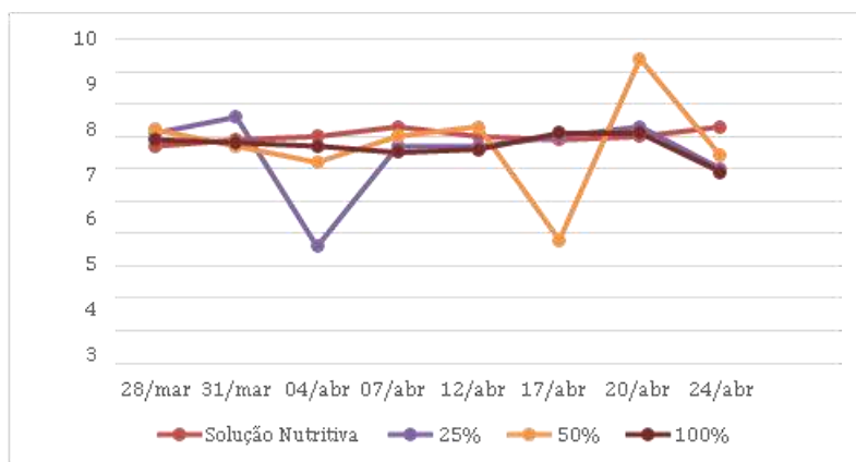
Figura 1. Variação do pH das diferentes soluções nutritivas utilizadas no experimento.
