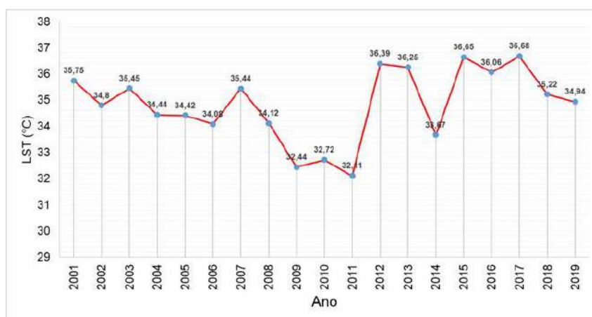
Figura 3. Série temporal da média anual de LST.
