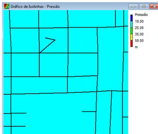
Figura 4. Pressão na rede - cenário 3.
