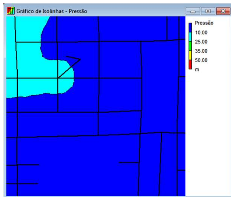
Figura 3. Pressão na rede - Cenário 1.
