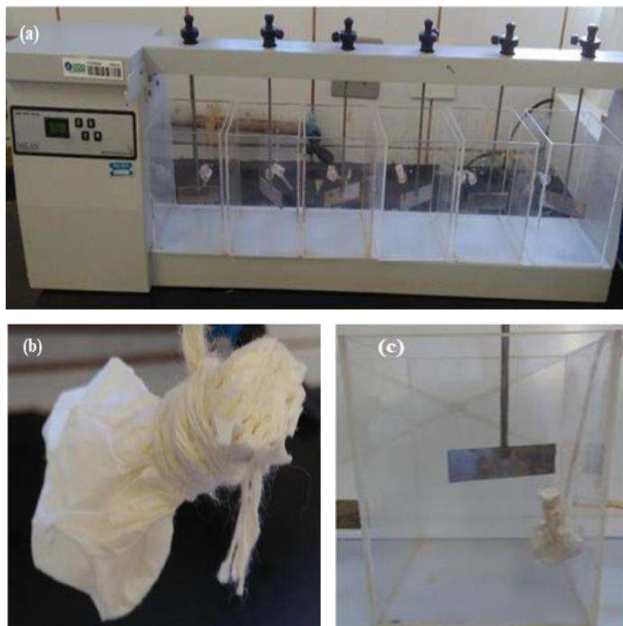
Figura 1. Aparelho Jarrest utilizado no procedimento experimental (a); saco confeccionado com papel filtro (b); Jarro com sacos fixados (c).
