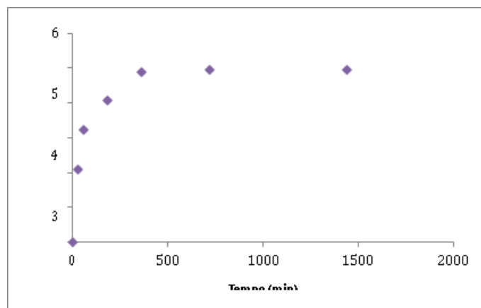
Figura 4. Adsorção de glifosato em filme de quitosana ( 5 \text{ mgL}^{-1} de glifosato pH 6, 25^{\circ}\text{C} ).
