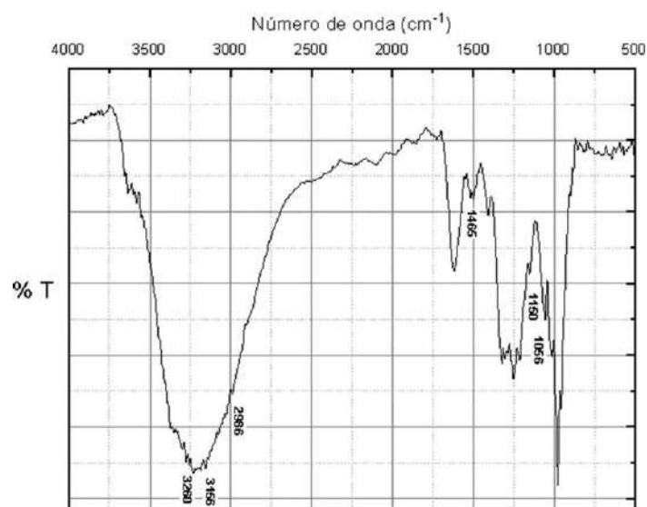
Figura 1. Espectro de absorção no infravermelho dos filmes de quitosana.
