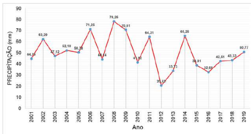
Figura 4. Série temporal da média anual de Precipitação.
