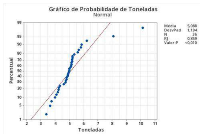
Figura 3. Teste de Normalidade.
