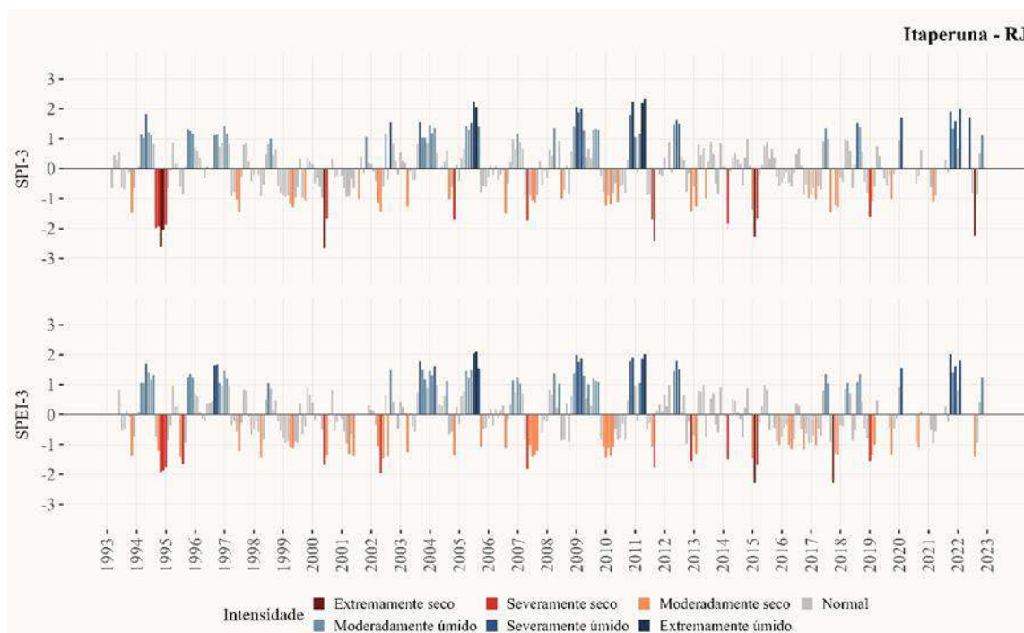
Figura 4. Séries temporais do SPI e SPEI de 3 meses para o município de Itaperuna-RJ, referentes ao período de 1993 a 2022.
