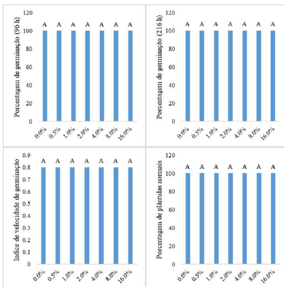
Figura 2. Parâmetros de germinação com (A) 96 horas, (B) 216 horas, (C) índice de velocidade de germinação e (D) plântulas normais.
