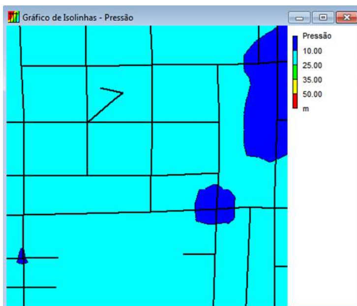
Figura 3. Pressão na rede - cenário 2.
